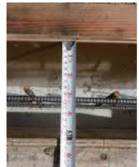
かぶり厚さ確認
